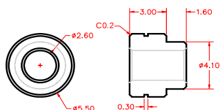
33- 72011- 0030
