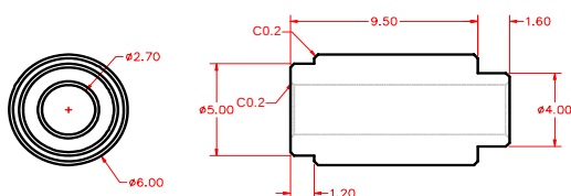
33- 72011- 9P50
