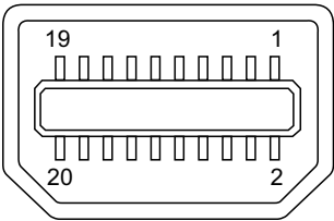
Figure 3-17: Mini DisplayPort Pin Definition
