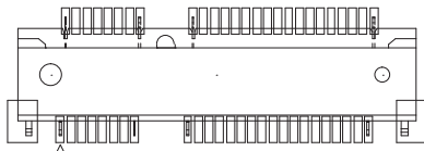
Figure 3-16: Mini PCIe Pin Definition
